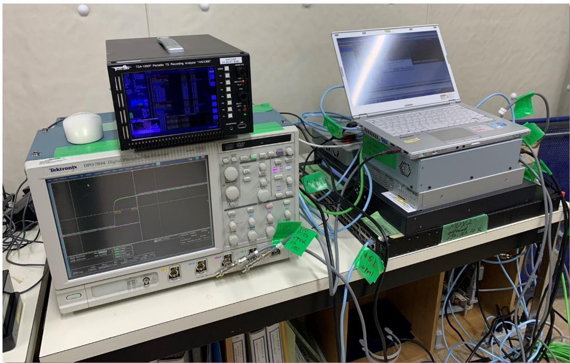
毎日放送 生駒送信所側
